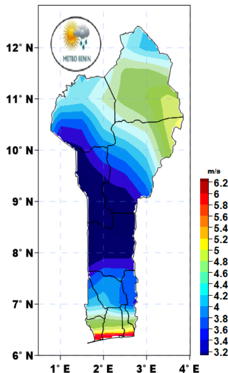
FIGURE 9 – Vitesse du vent maximal instantané.
