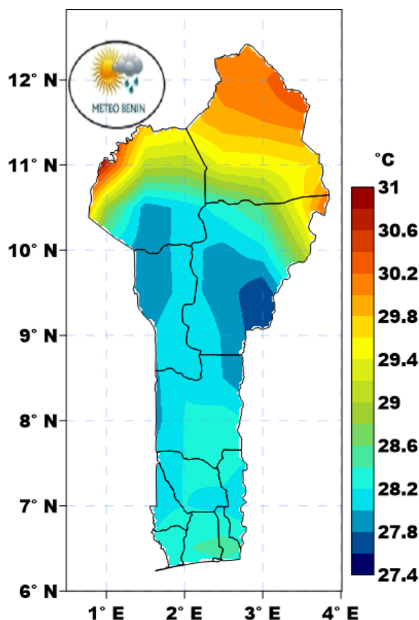
FIGURE 5 – Température moyenne mensuelle Novembre
