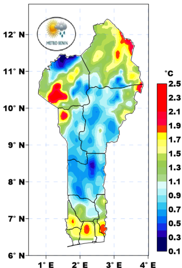
FIGURE 6 – Ecart à la normale de la température moyenne
