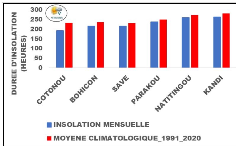
FIGURE 7 – Cumul mensuel d'insolation de mois de Novembre 2024 comparée à la normale
