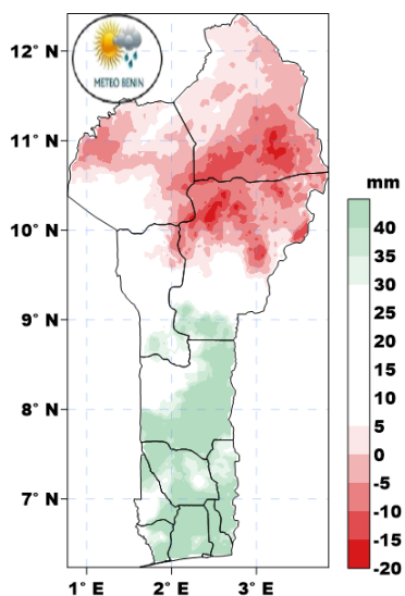
FIGURE 4 – Anomalie des précipitations
