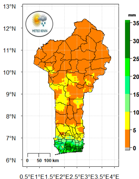
FIGURE 3 – Cumul mensuel de pluie
