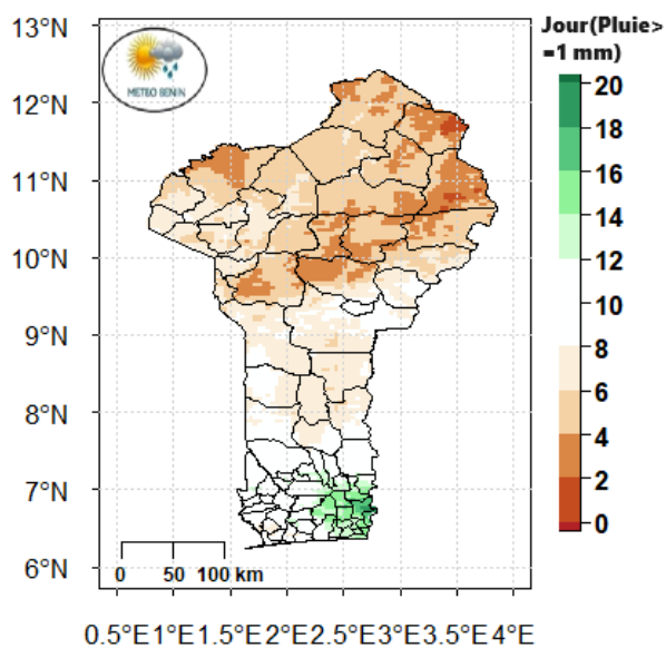
FIGURE A1 – Nombre de jours de pluies
