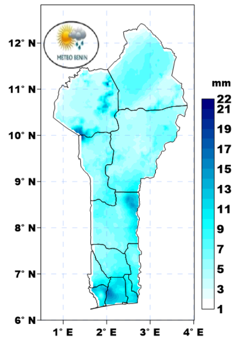
FIGURE A2 – Pluies maximales journalières
