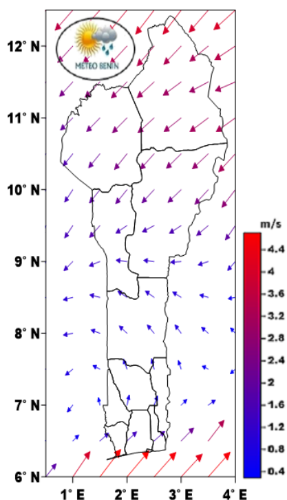
FIGURE 8 – Direction et vitesse du vent moyen.
