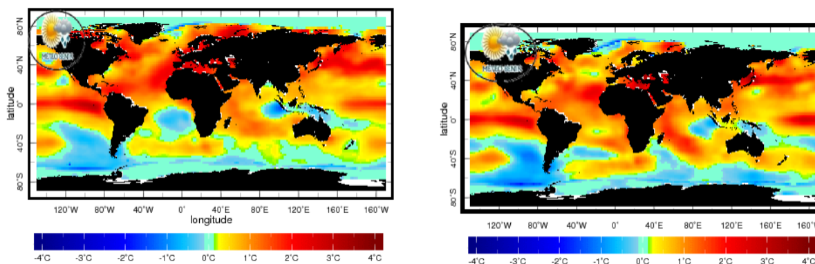
FIGURE 2 – Anomalies de température de surface des océans au cours des mois d'Octobre (à gauche) et Novembre (à droite) (NOAA/NCDC)
