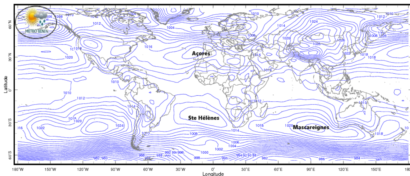
FIGURE 1 – Pression réduite au niveau de la mer (hPa), Moyenne de Novembre 2024
